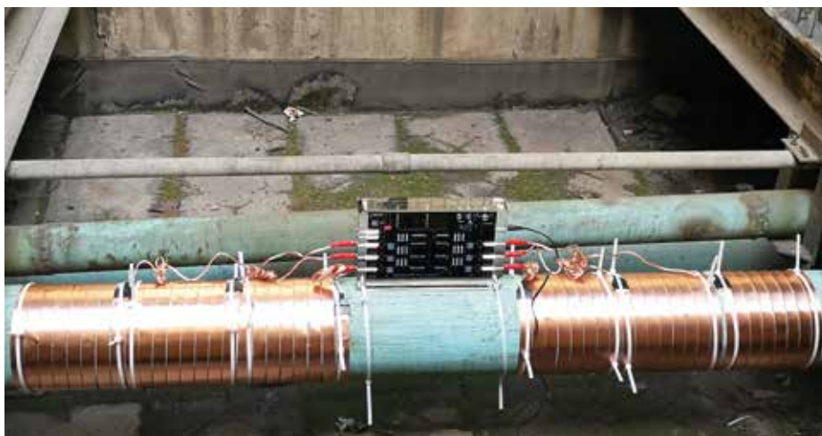
Vulcan S100 安装在华能大连电厂中冷却塔的进水管道上，管道直径是150mm，管道材质是钢管
