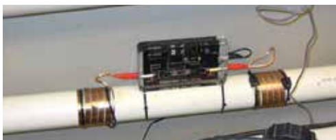
安装在泳池撇沫器主管线上的Vulcan 5000
