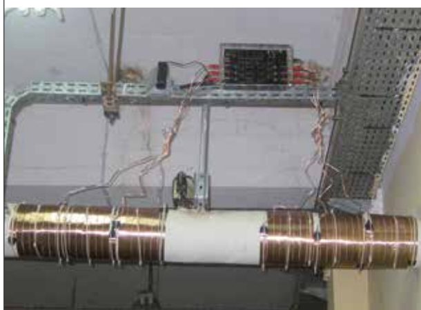
Vulcan S100 和 Vulcan S250 物理水处理
