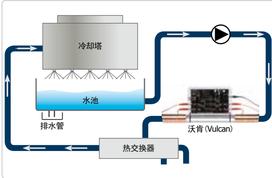
开路举例
